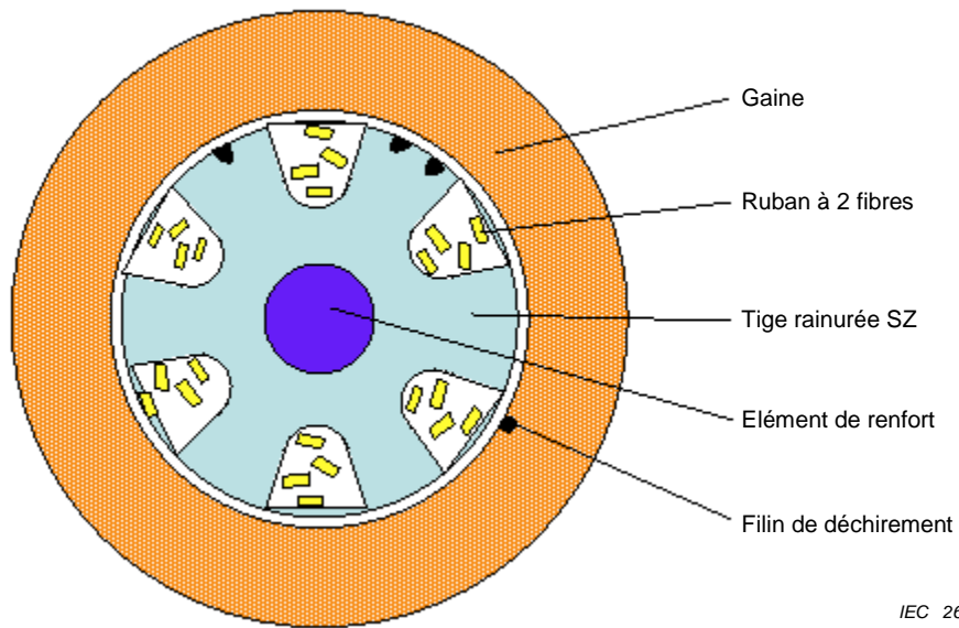
Figure A.6 – Exemple de coupe transversale d’un câble intérieur de type à jonc rainuré SZ (disposition en hélice croisée) avec rubans à 2 fibres
